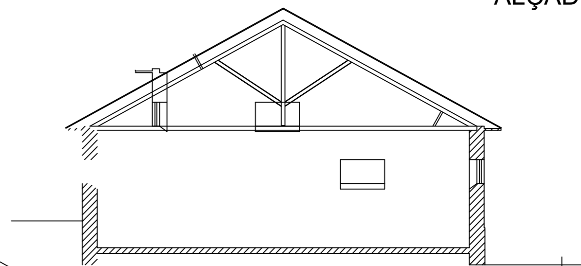
CORTE E/F
