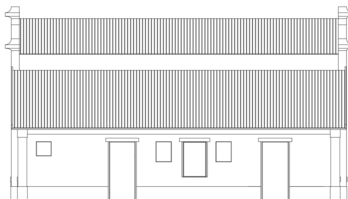
ALÇADO SUL
