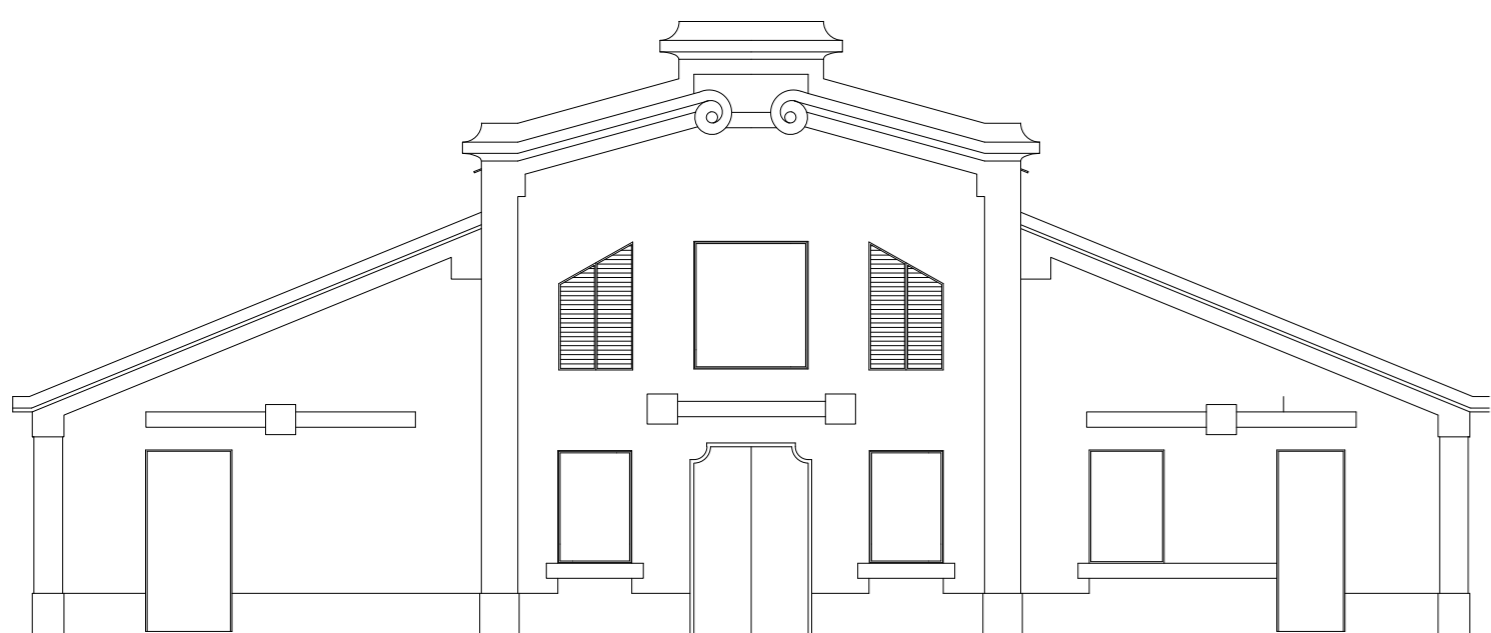
ALÇADO NASCENTE
